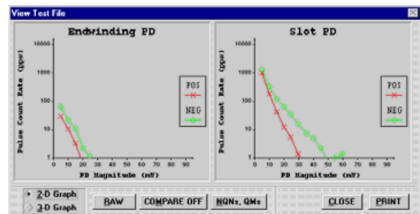
Grafico per l'analisi dell'altezza degli impulsi scariche parziali positive e negative
